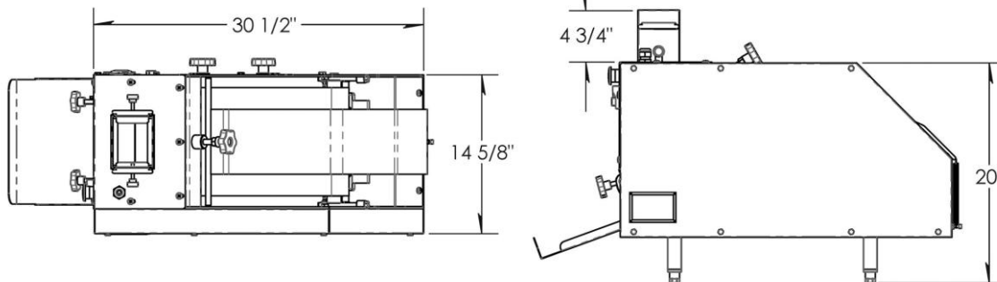
POCO MOULDER dimensions
